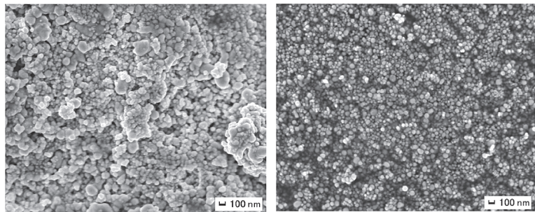
図7 銀粉分級前後のSEM写真比較
